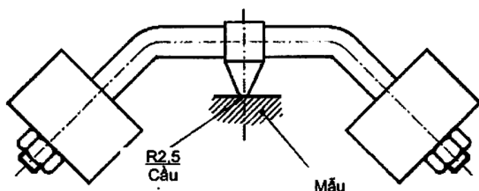
Hình 5 – Thiết bị thử ép viên bi
