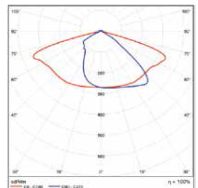
Sơ đồ phân bố ánh sáng phù hợp với các loại tuyến đường
