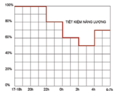
Sơ đồ Dimming 5 cấp theo thời gian
